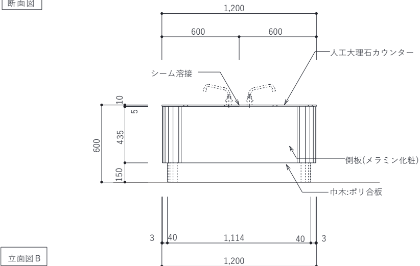
断面図
