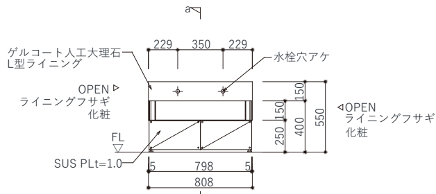
立面図
