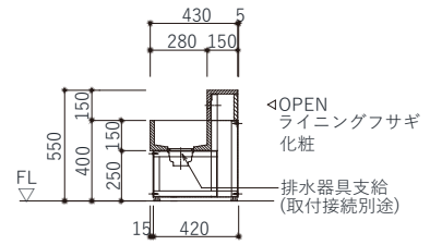
a-a断面図
