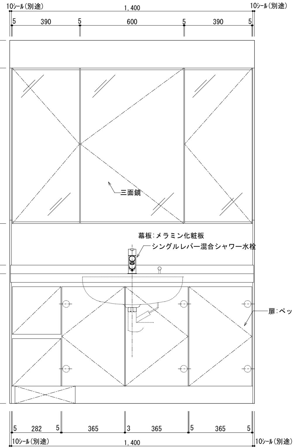
立面図
