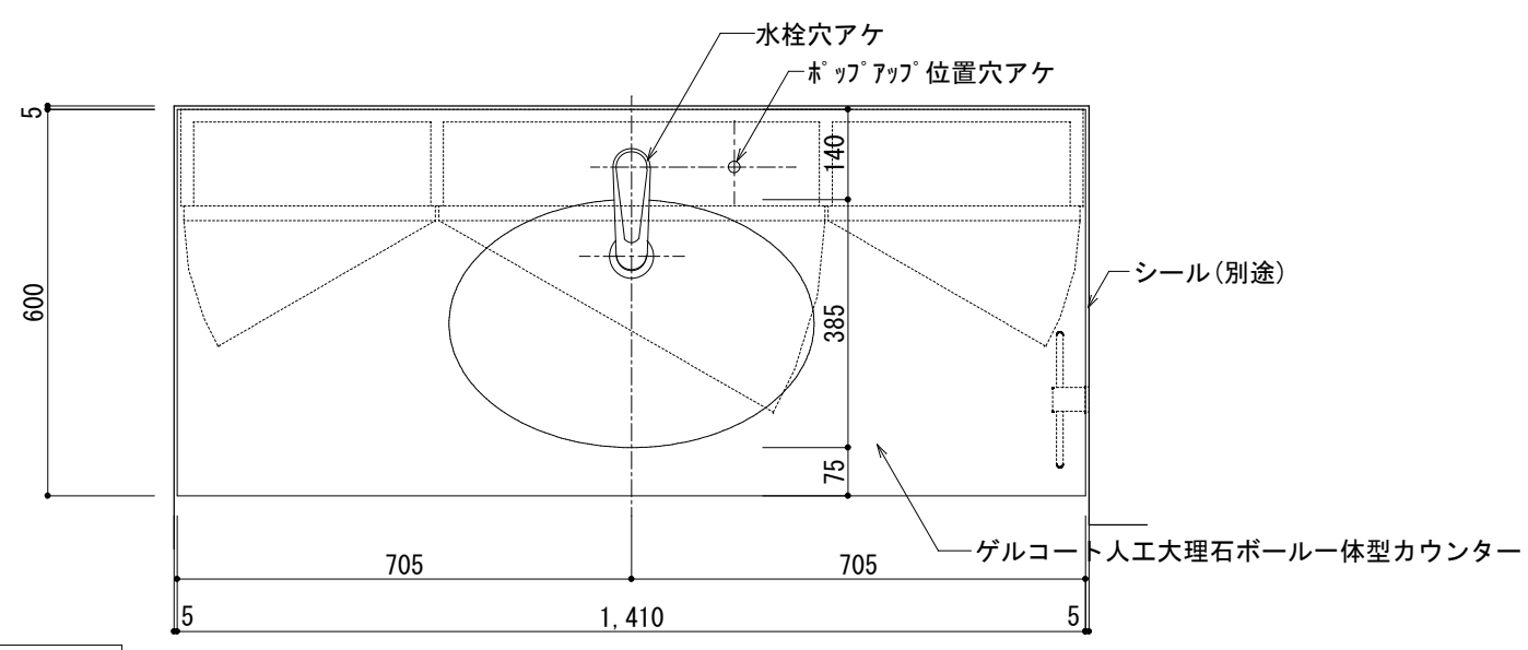
平面図
