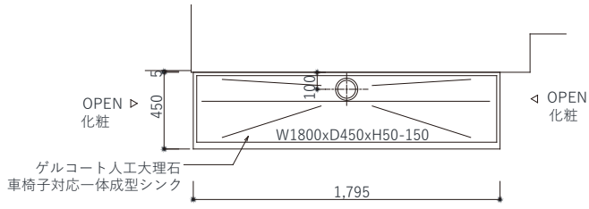
平面図
