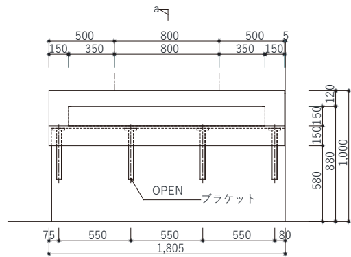
立面図
