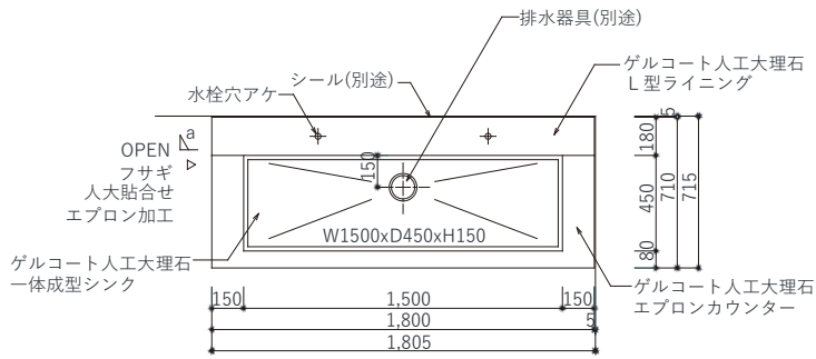
平面図
