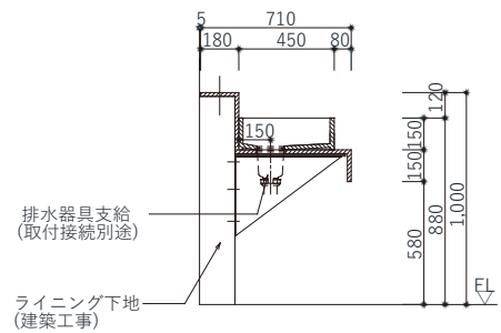
a-a断面図
