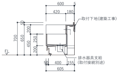
a-a断面図
