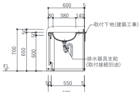
c-c断面図
