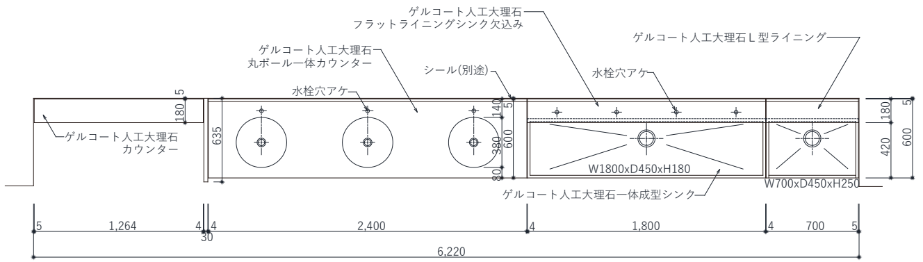
平面図
