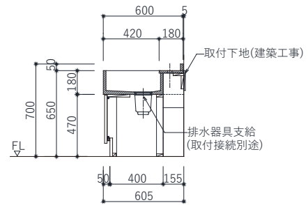
b-b断面図
