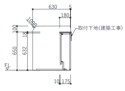
d-d断面図
